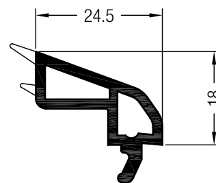
Glasleiste 24,5 Softline
