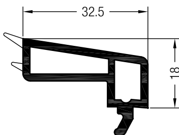
Glasleiste 32,5
