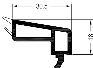
Glasleiste 30,5
