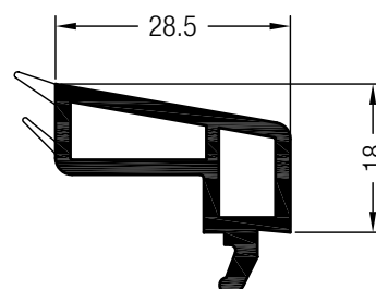
Glasleiste 28,5
