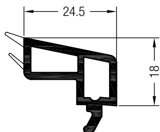
Glasleiste 24,5
