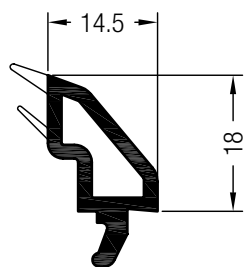
Glasleiste 14,5 Softline
