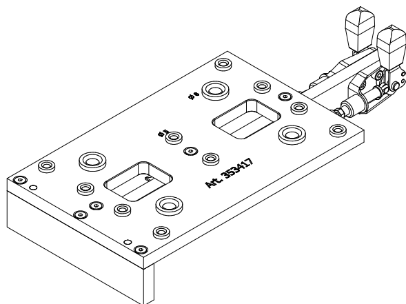
Bohrschablone 1353417
