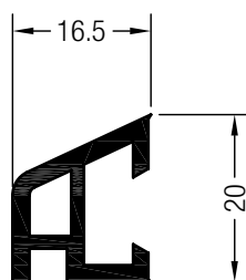
Wetterschenkel Nr. 3
