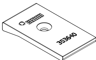
Schraubstück Zink-Druckguss
