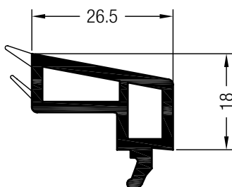
Glasleiste 26,5
