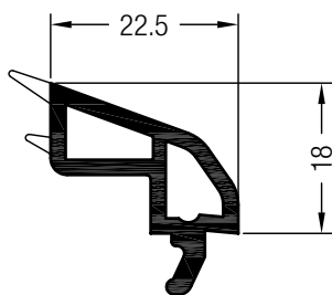
Glasleiste 22,5 Softline
