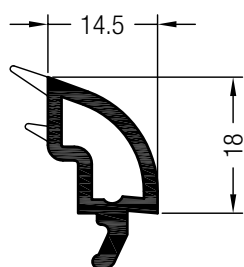
Glasleiste 14,5 rund
