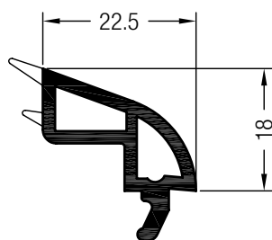
Glasleiste 22,5 rund
