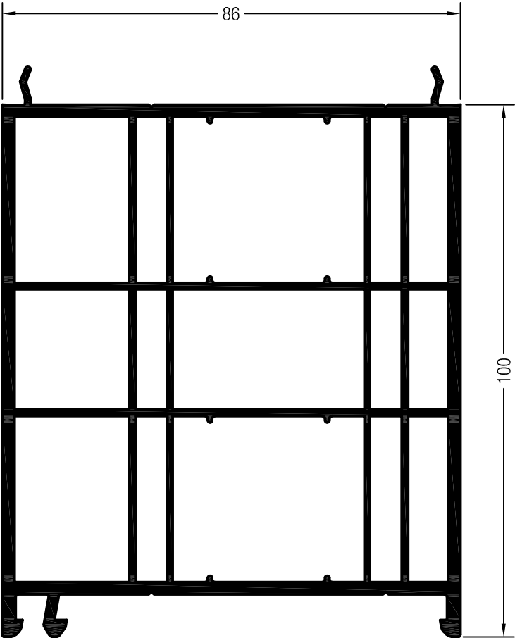
Blendraahmenverbreiterungen
