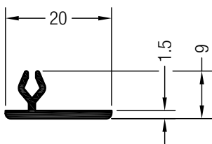
Füllprofil Nr. 2 für Silikonfuge
