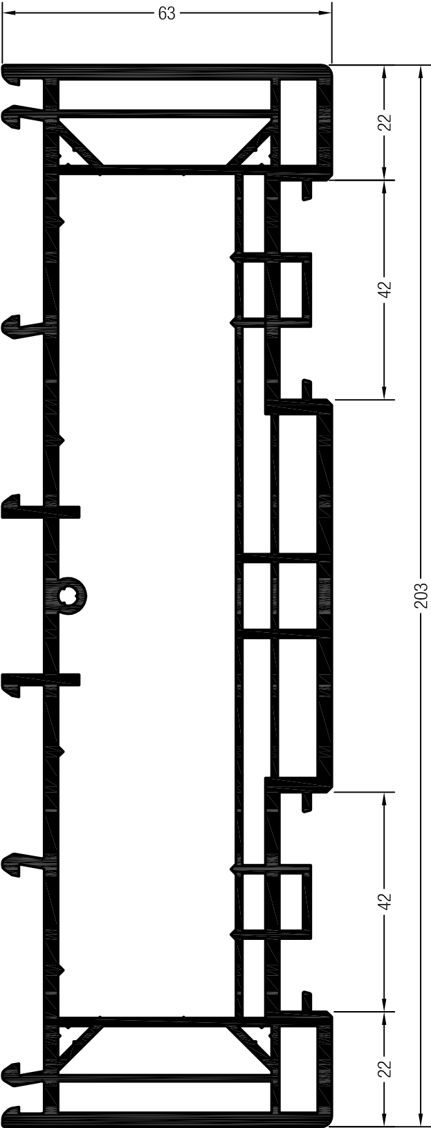
Zargenprofile
