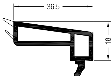
Glasleiste 36,5
