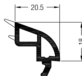
Glasleiste 20,5 rund
