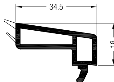
Glasleiste 34,5
